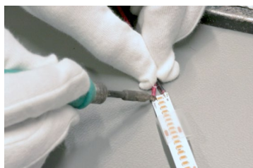
Konfektionierung LED-Flexbänder
