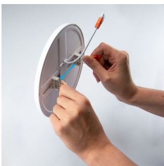
Variabler Lochausschnitt
